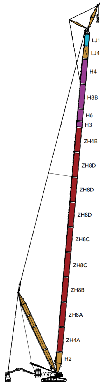
ZHJFJDB (102m+12m)~(165m+12m)
